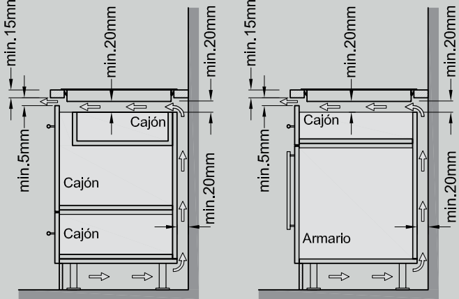
Sơ đồ lắp đặt cho bếp cảm ứng
