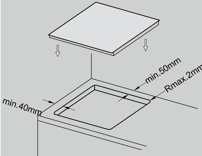
Kiểm tra kích thước lỗ đặt của từng loại bếp
