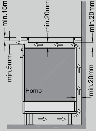
Khoảng cách tối thiểu cho hệ thống thông gió.
