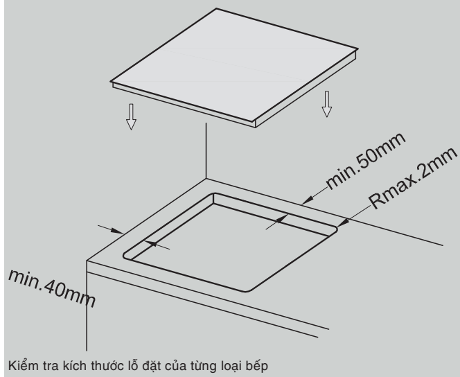
Khoảng cách tối thiểu của lỗ đặt bếp đến tường
